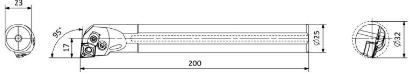
AKKO® A25R PCLNR 12C
