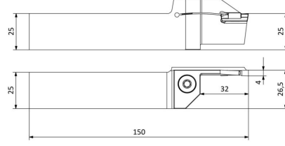
AKKO® AAKT-IG-L-2525-110-200-4-T32
