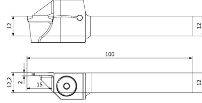
AKKO® ADKT-K-L-1212-2-T15
