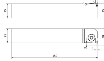
AKKO® ALKT-ZCC2-L-2525-35-...-3-T4
