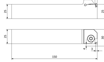
AKKO® ALKT-ZCC2-L-2525-35...-3-T4
