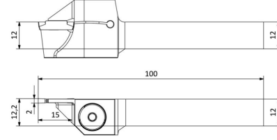
AKKO® ADKT-K-L-1212-2-T15
