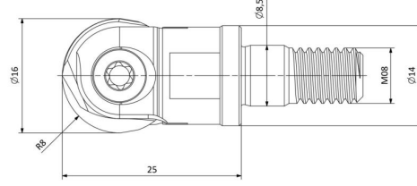
AKKO® APMR-P3216-D16-M08-L25
